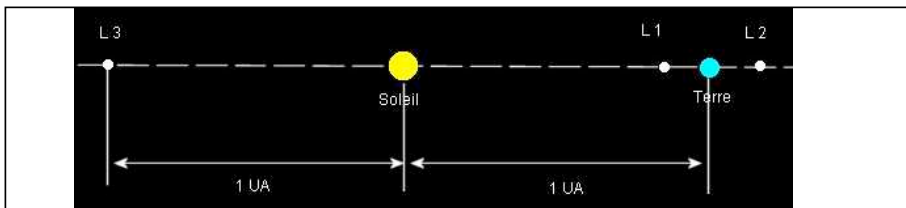
Positions des points L1 à L3 sur l'axe Soleil-Terre
