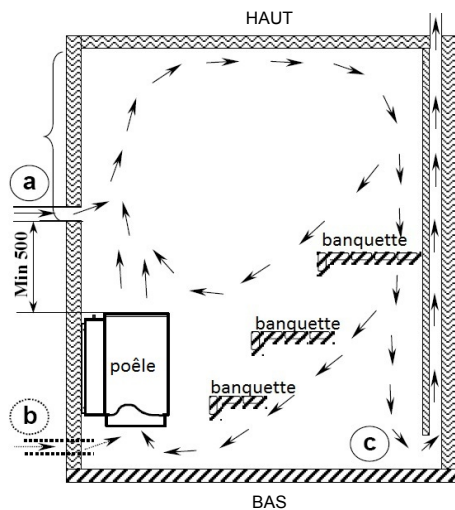
Vue en coupe verticale du sauna
