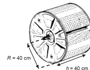
Figure 2. Schéma du tambour du lave-linge
