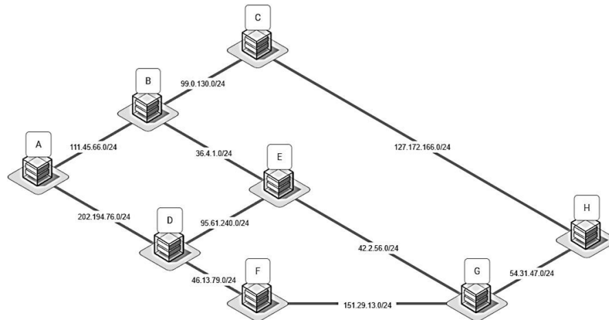
Figure 1. Réseau de routeurs
