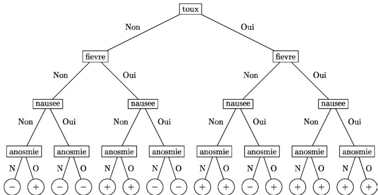
Figure 1. Exemple d'arbre de décision binaire
